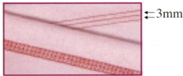
三本縫(3針4線)
